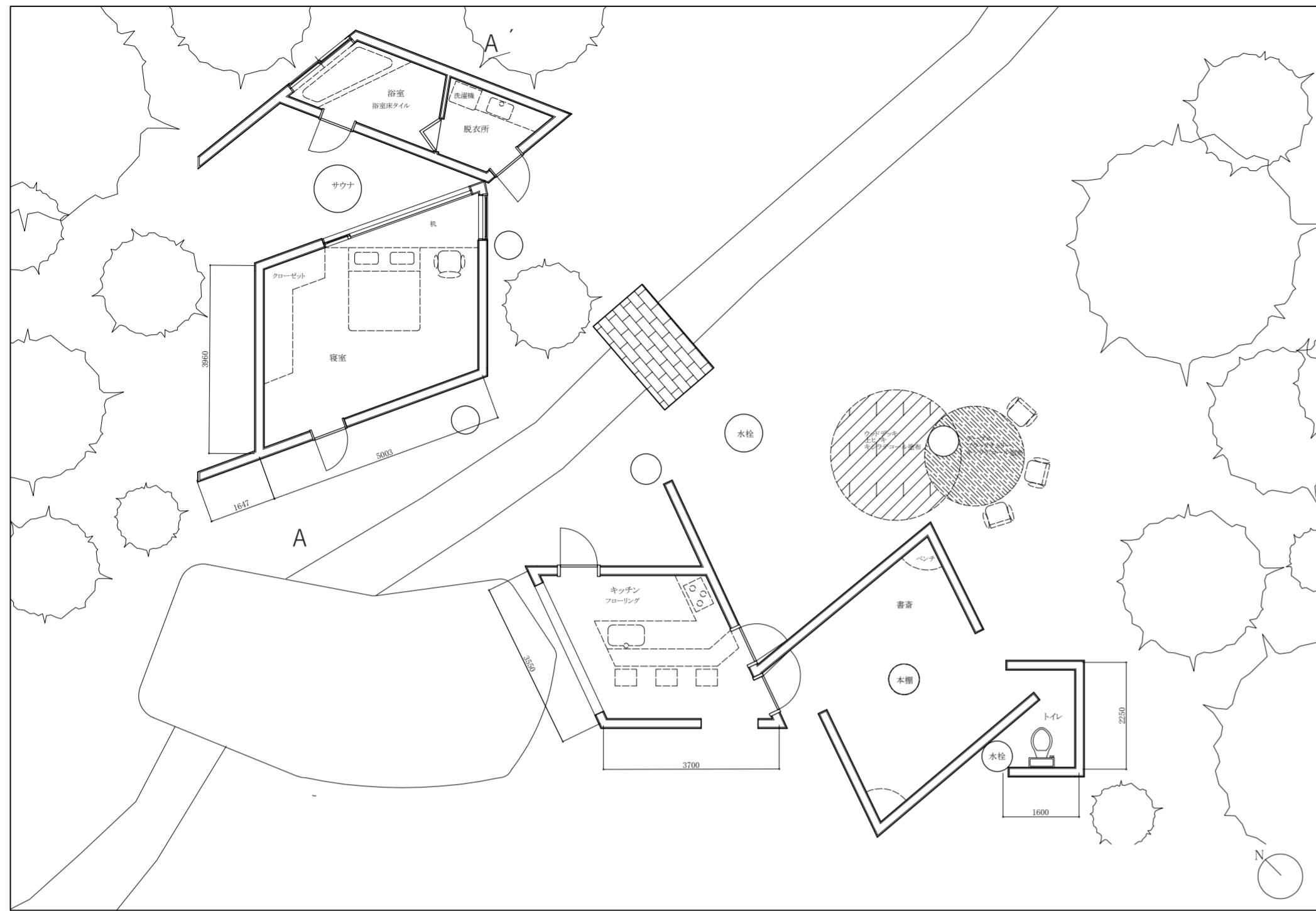
1/100 平面図
