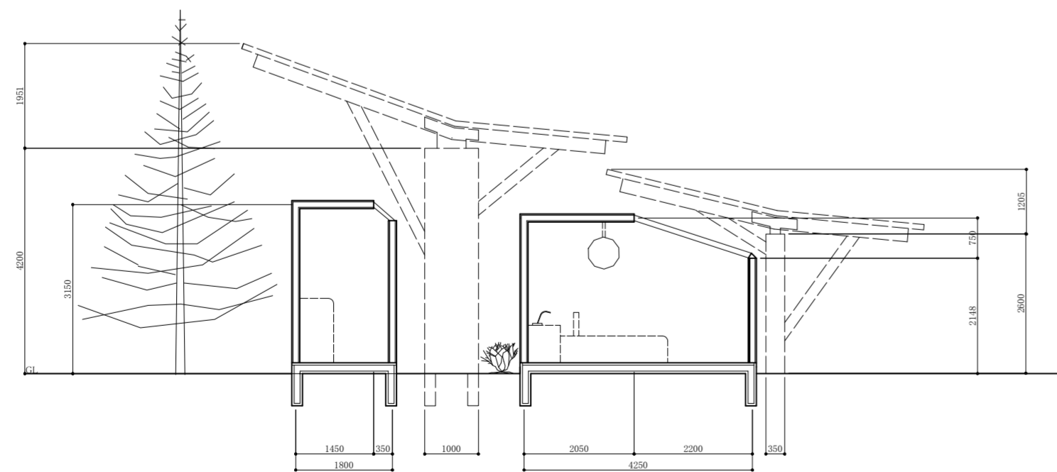
1/100 断面図
