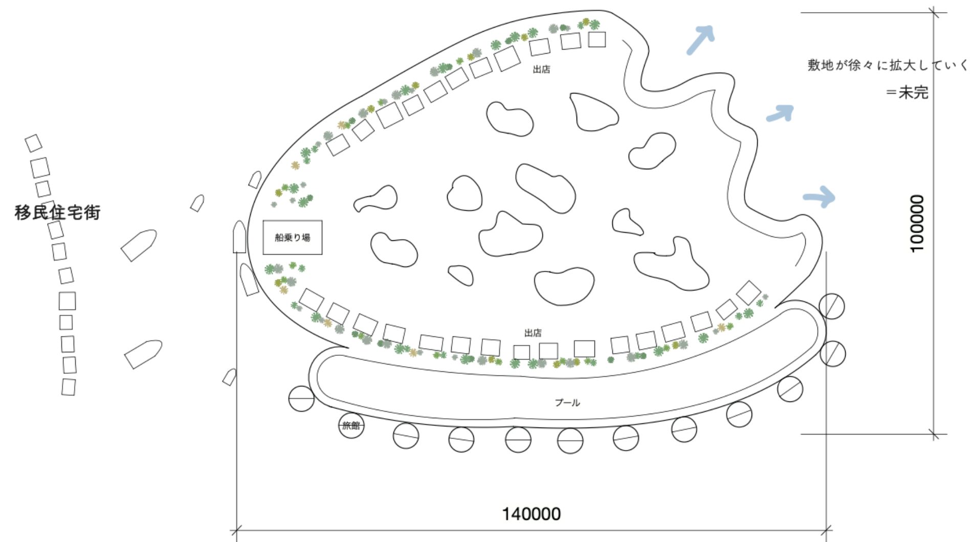
LOTUS ISLAND 平面図 S=1:100
