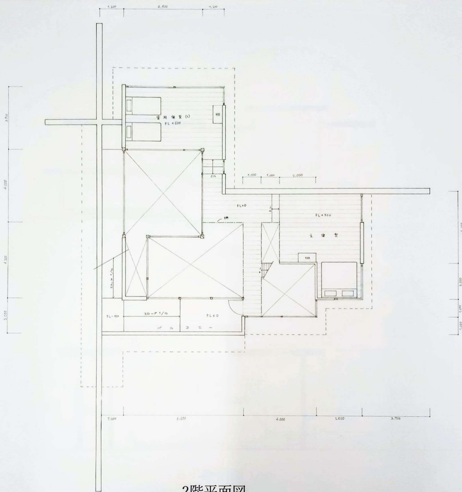
2階平面図
