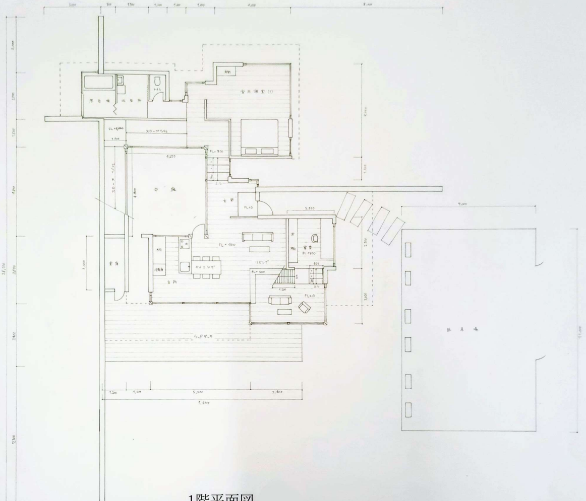
1階平面図
